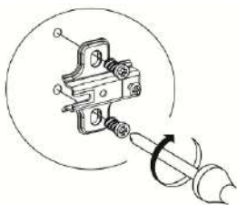
Рис.1 Монтаж крестовины петли на боковину
