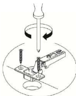
Рис.2 Монтаж чашки петли на фасад
